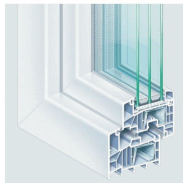
OKNA ENERGOOSZCZĘDNE 88 PLUS
